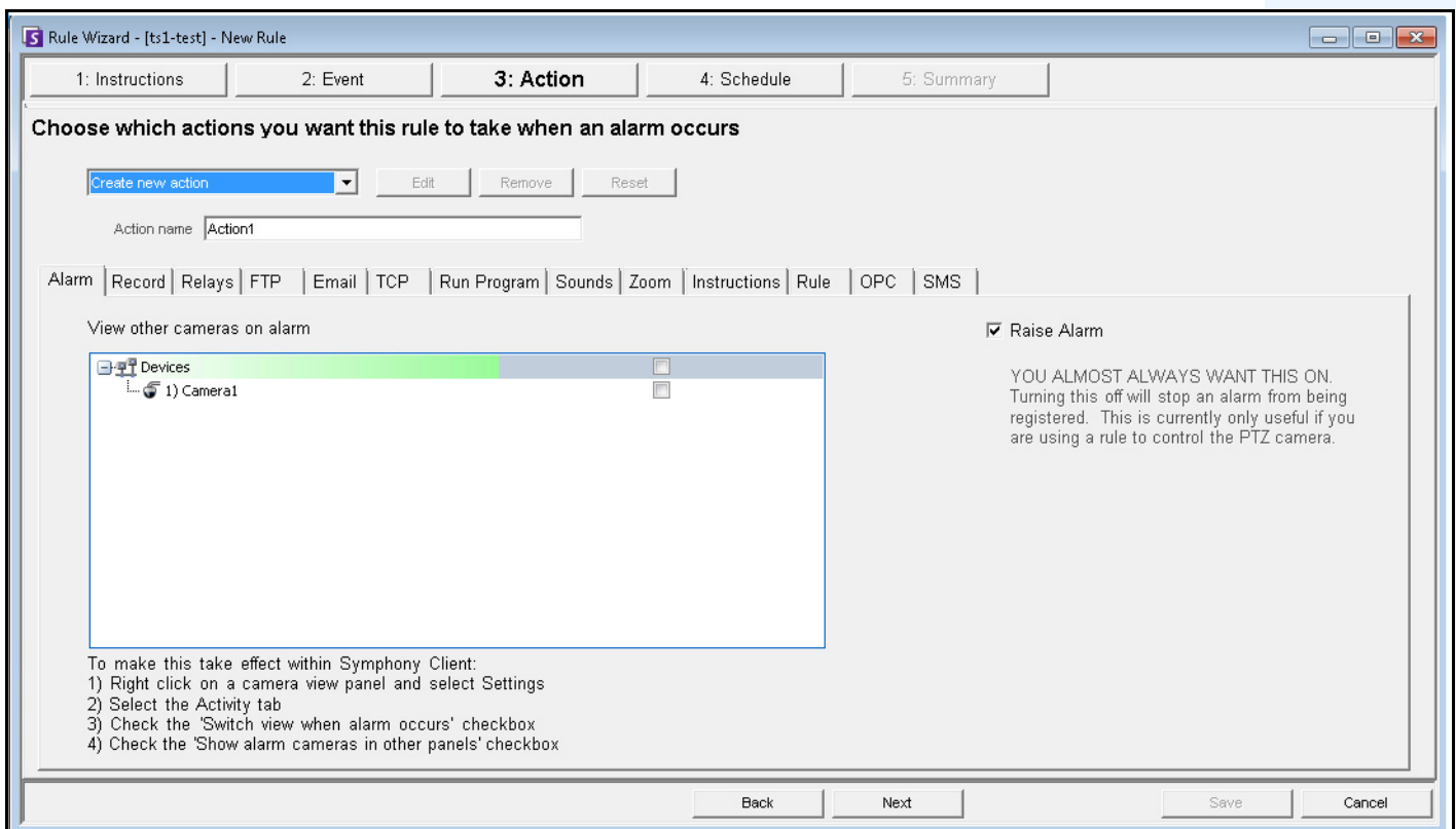
图 34. 规则向导 - 操作
