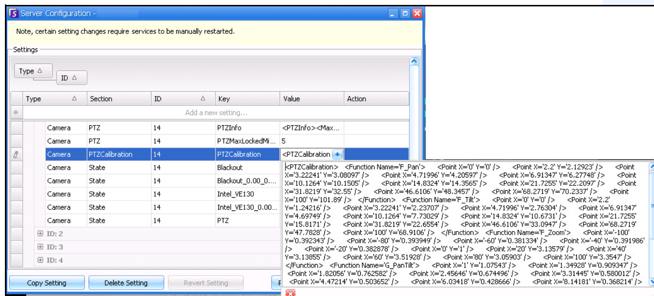
图 32. 复制“PTZ Calibration Value”（PTZ 校准值）字段中的内容
