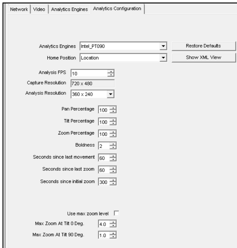
图 27. 选择 Intel_PT090 引擎时的“分析配置”选项卡
