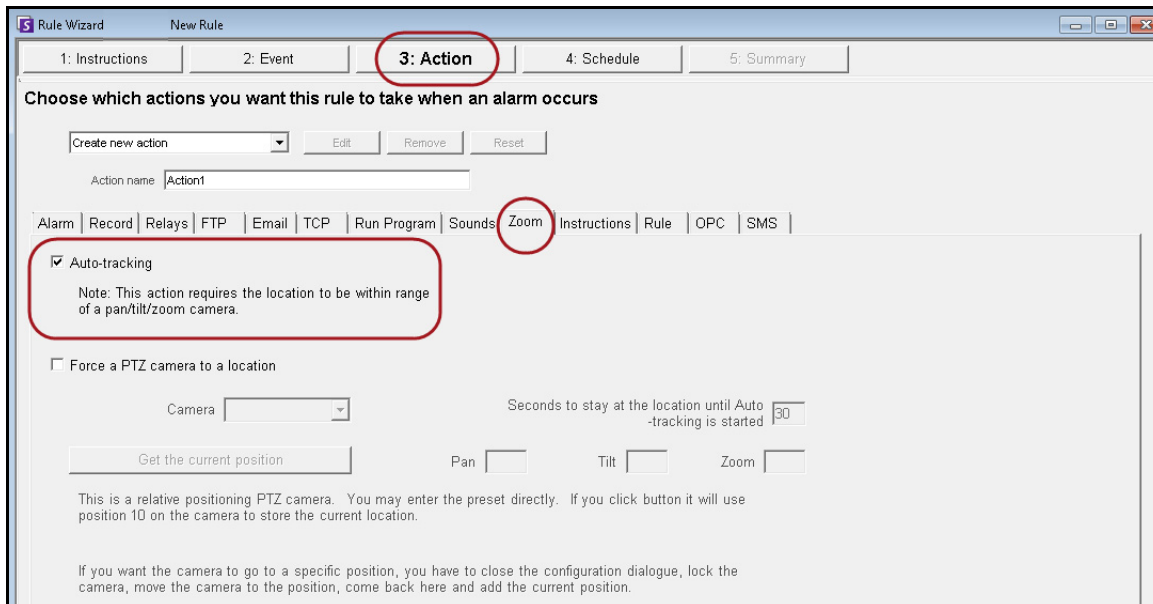
图 30. 选中“缩放”选项卡中的“自动跟踪”选项
