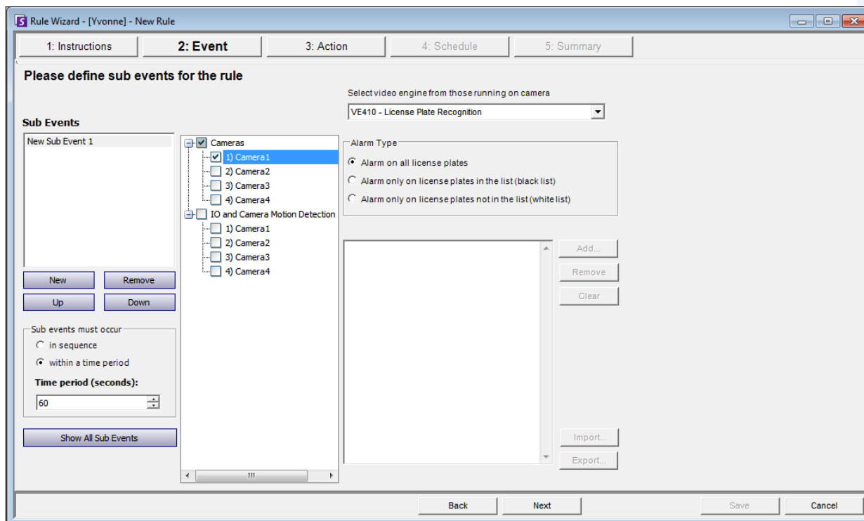
图 33. “License Plate Recognition”（牌照识别）的“规则向导 - 事件”选项卡
